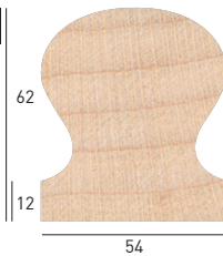
Handlauf Main courante
